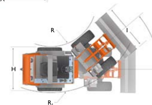
Dimensions avec cabine ROPS
