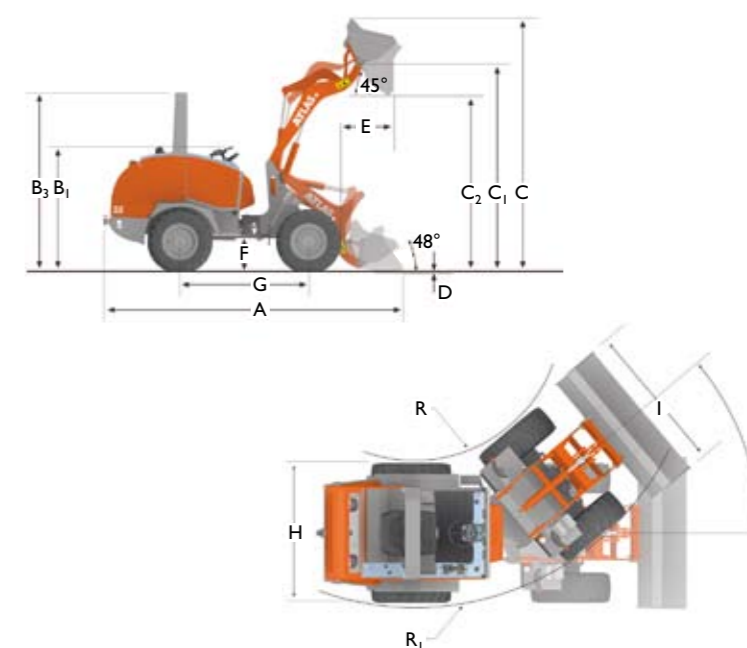
Dimensions avec cabine ROPS
